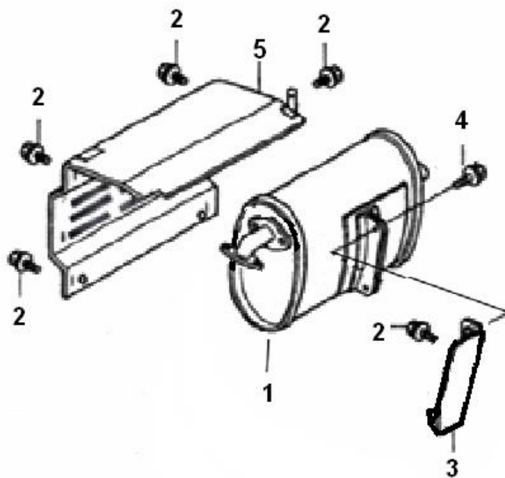
マフラー (MUFFLER)
