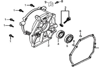
クランクケースカバー (CRANKCASE COVER)
