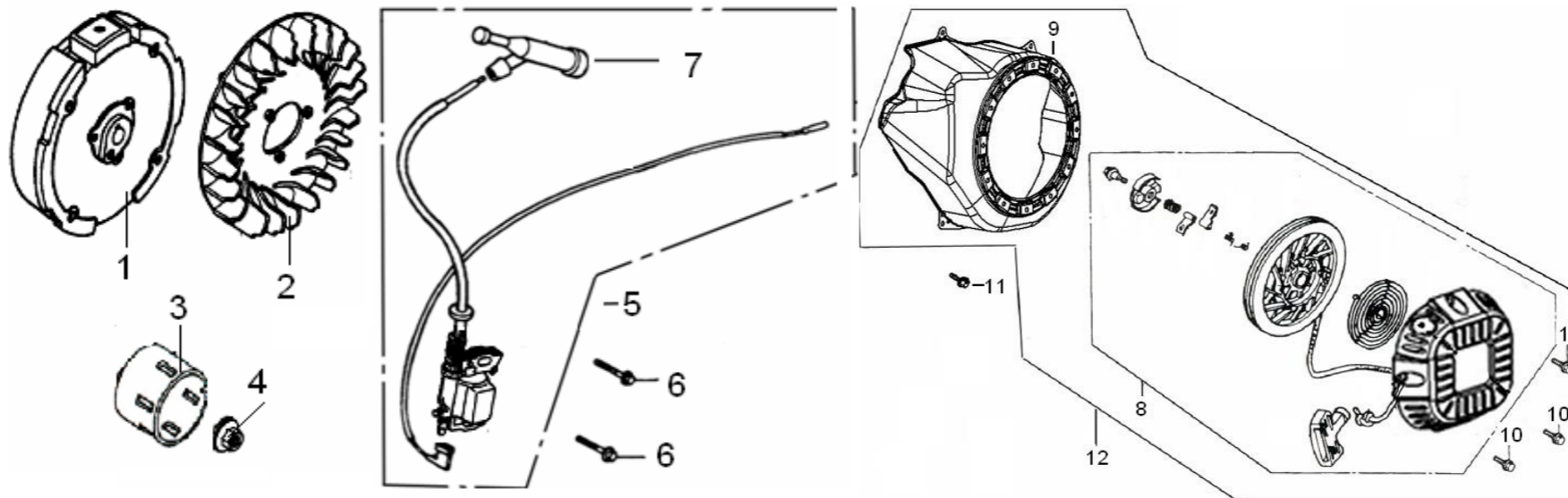
スターター/点火システム (STARTER/IGNITION ASSY.)
