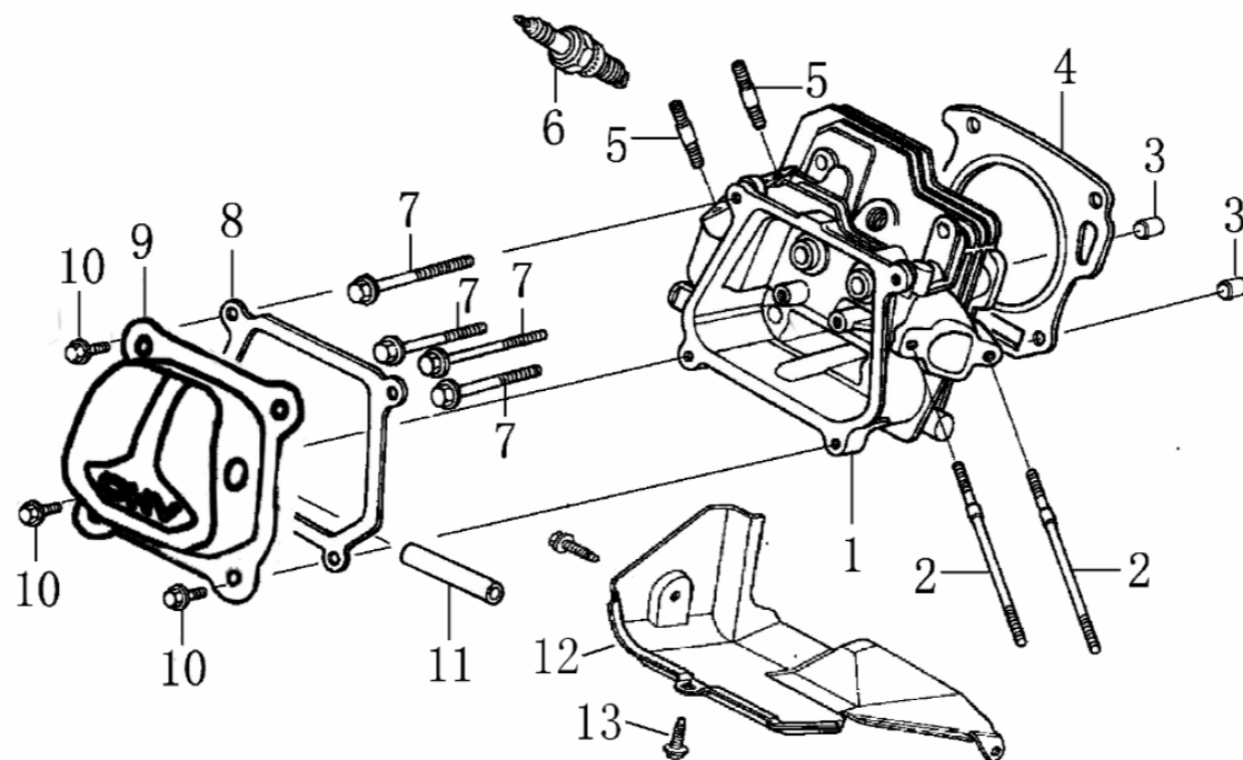
シリンダーヘッド (CYLINDER HEAD)
