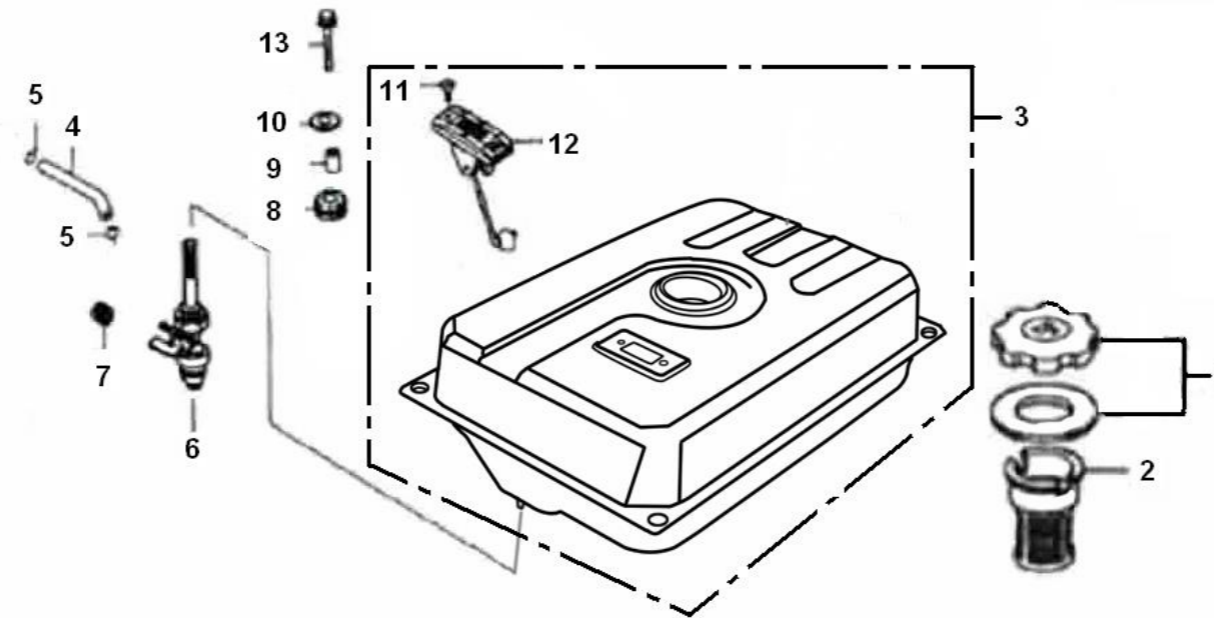
燃料タンク (FUEL TANK)
