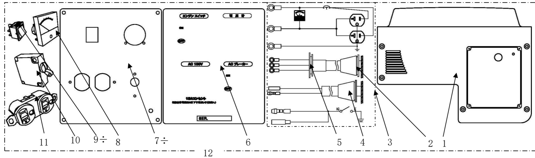
コントロールパネル (CONTROL PANEL ASSY.)
