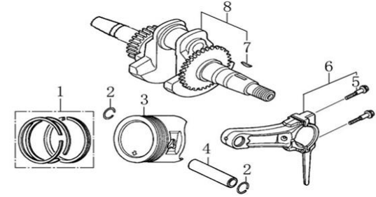
クランクシャフト/ピストン (Crankshaft_Piston)
