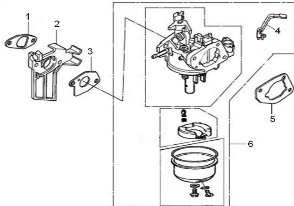
キャブレター (CARBURETOR)
