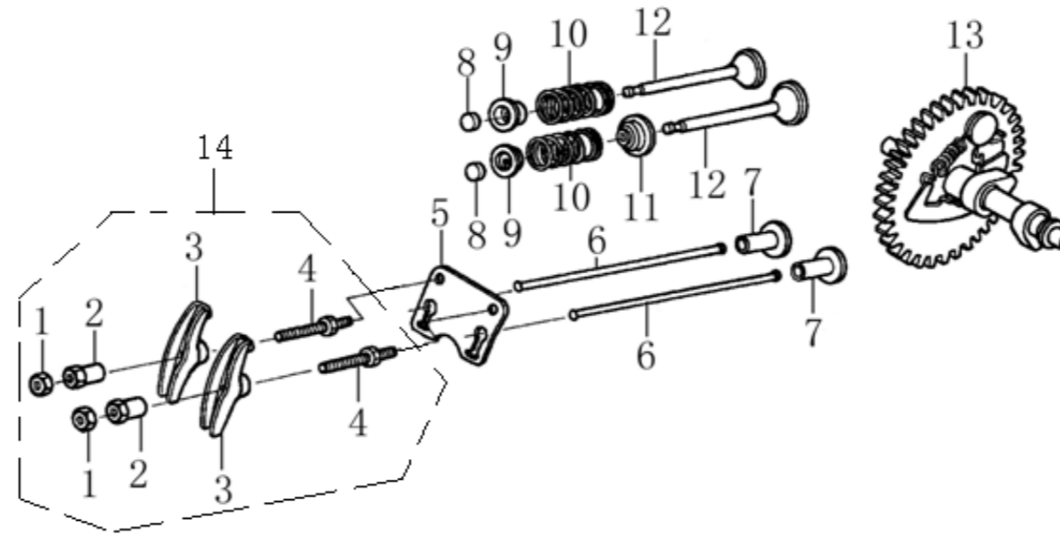
ロッカー/カムシャフト (ROCKER/CAMSHAFT)
