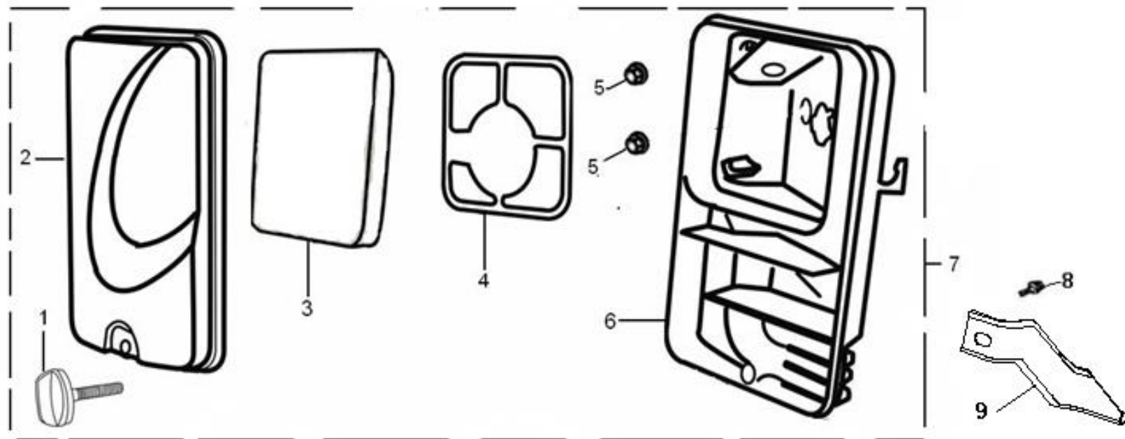
エアークリーナー (AIR CLEANER)
