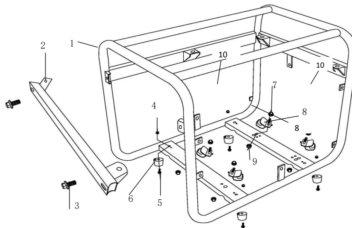
フレーム (FRAME)
