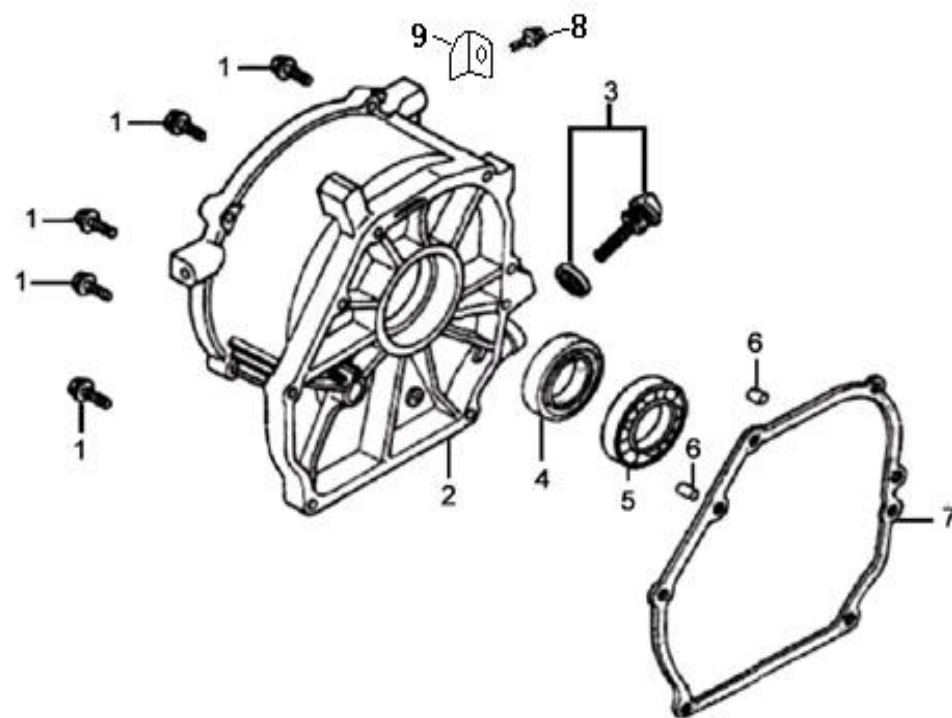
クランクケースカバー (CRANK CASE COVER)
