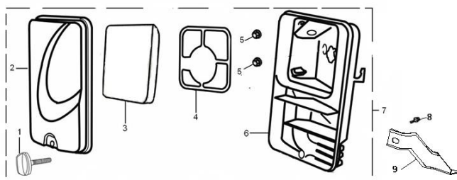
エアクリナー (AIR CLEANER)
