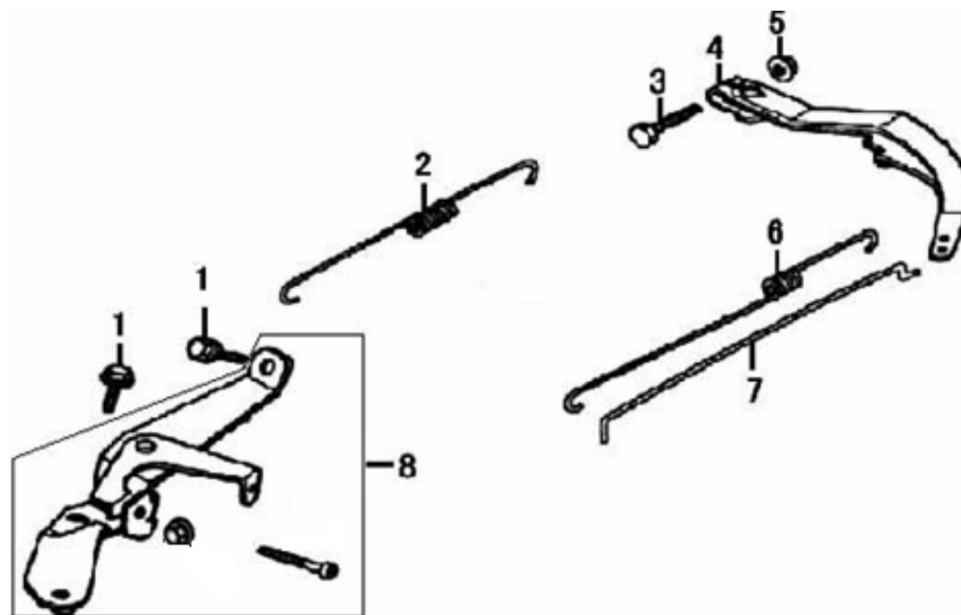
コントロール (CONTROL SYSTEM)
