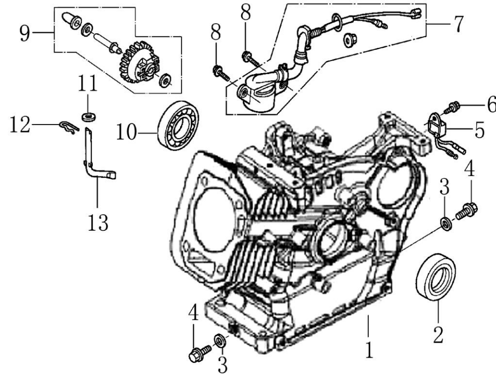
クランクケース (CRANK CASE)
