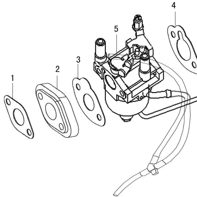
HPG1600i2 キャブレター (CARBURETOR ASSY)
