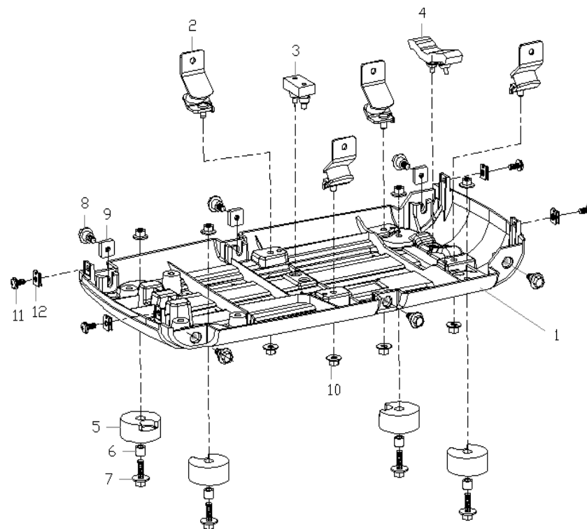
HPG1600i2 フレーム(FRAME)
