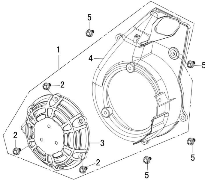
HPG1600i2 スターター(STARTER SUBASSEMBLY)
