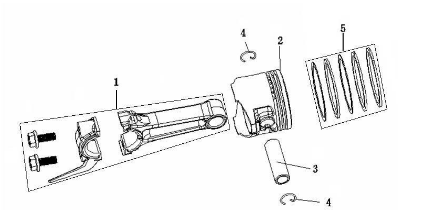
HPG1600i2 ピストン／コンロッド(PISTON/ROD ASSY .,CONNECTING )
