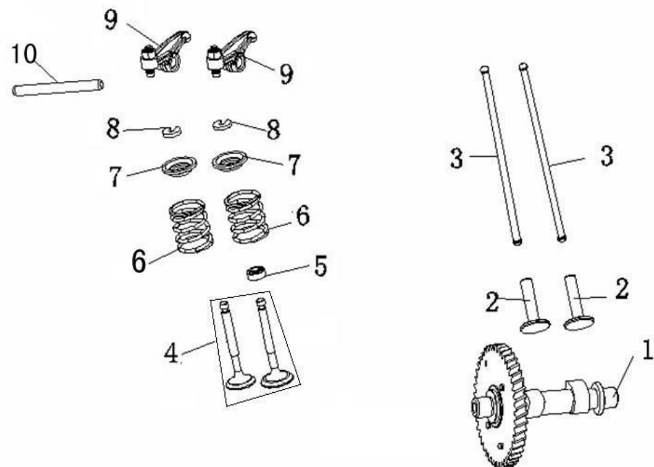
HPG1600i2 カムシャフト(CAMSHAFT)
