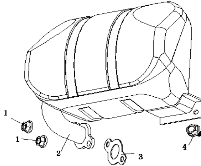
HPG1600i2 マフラー(MUFFLER ASSY)
