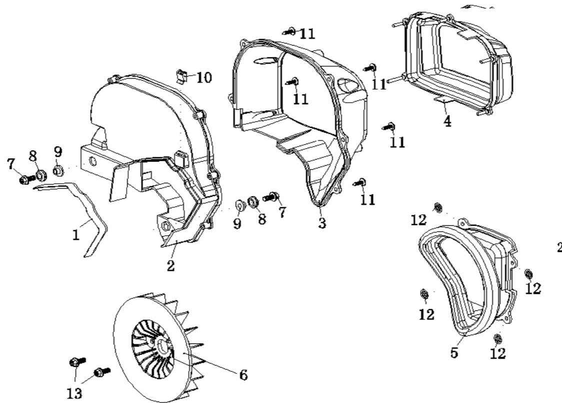
HPG1600i2 冷却システム
