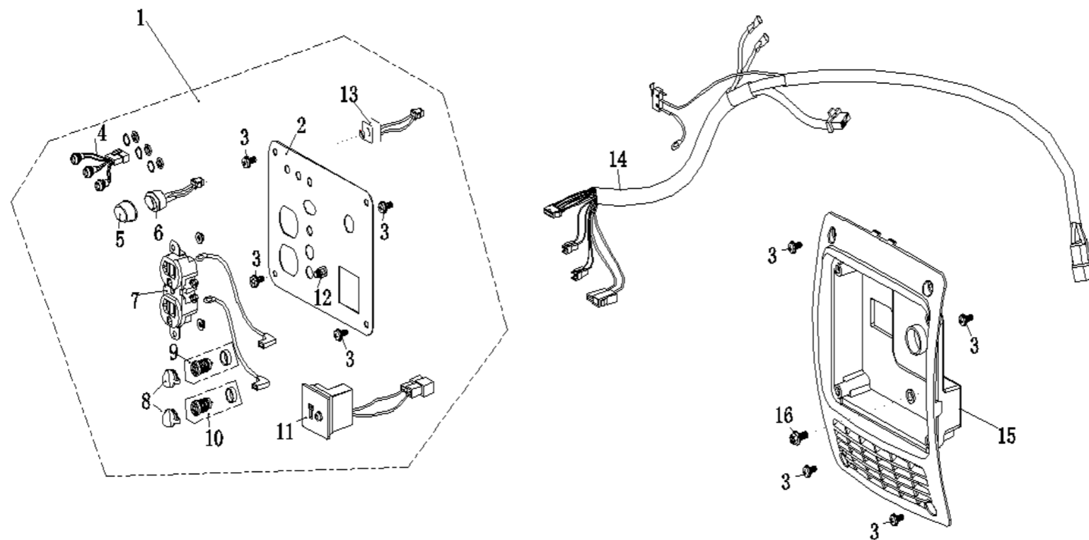
HPG1600i2 コントロールパネル (CONTROL PANEL)
