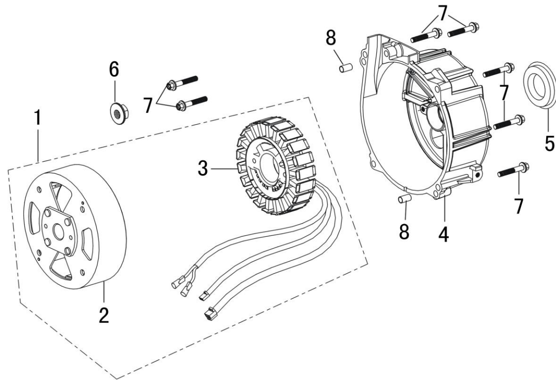
HPG1600i2 発電体 (ROTOR. STATOR)
