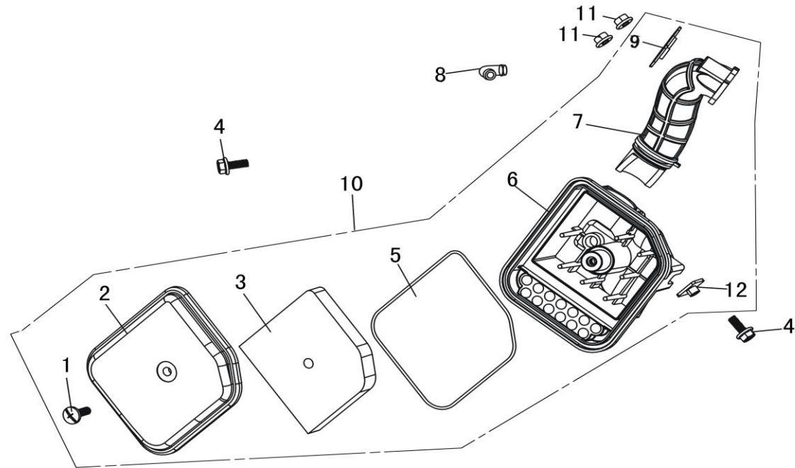
HPG1600i2 エアークリーナー (AIR CLEANER ASSY)
