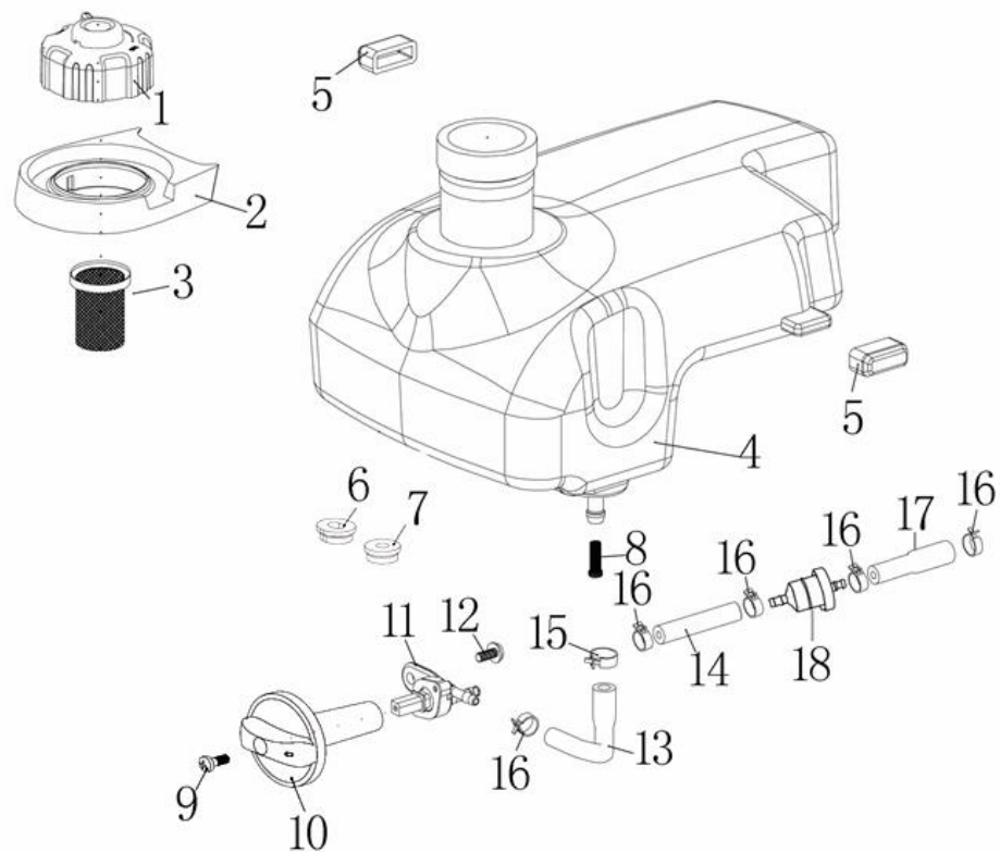
HPG1600i2 燃料タンク(FUEL TANK) (2)
