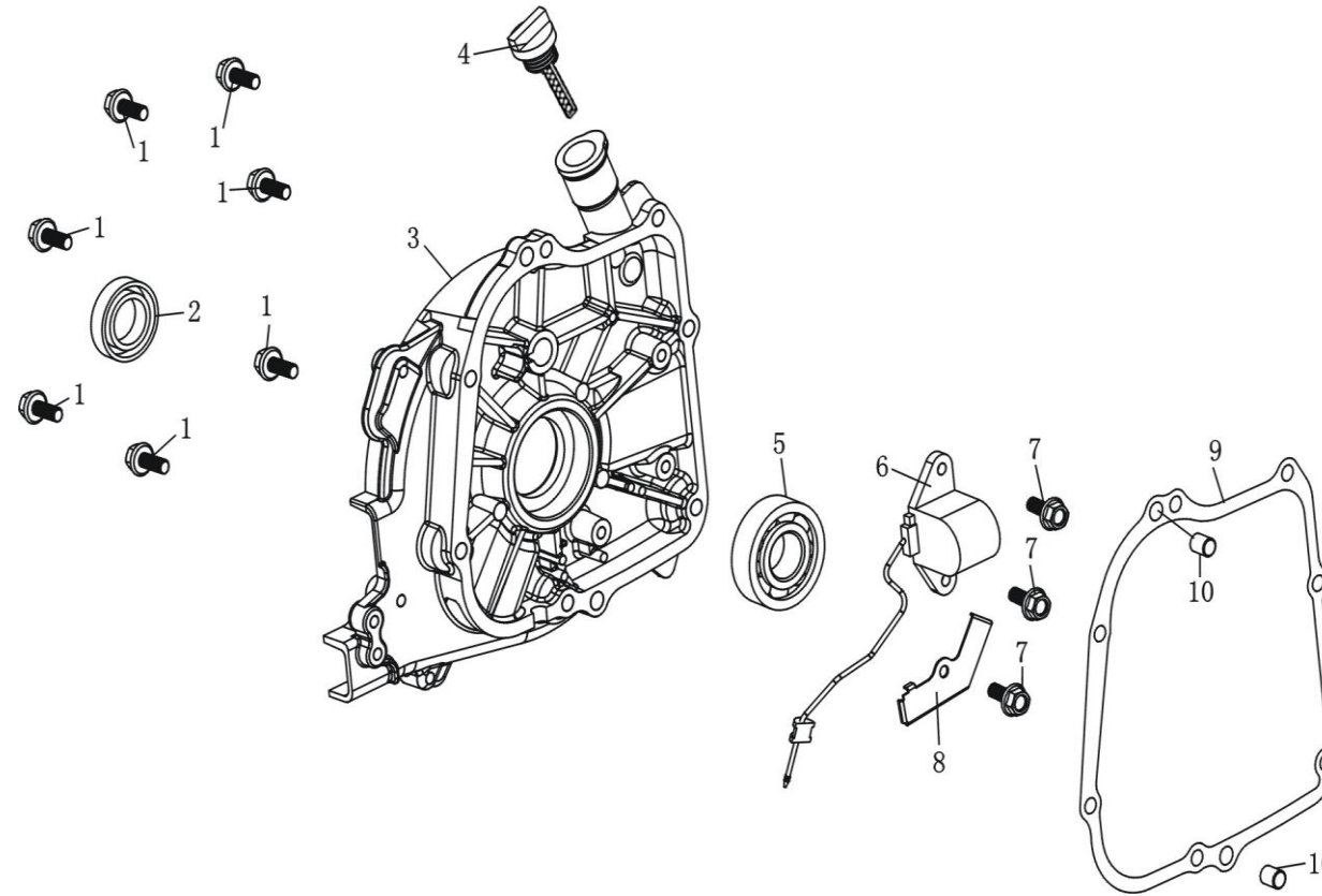
HPG1600i2 クランクケースカバー (CRANKCASE COVER)
