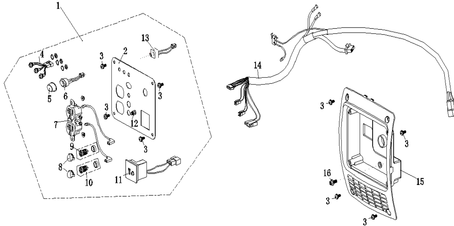
HPG1600i2 コントロールパネル (CONTROL PANEL)
