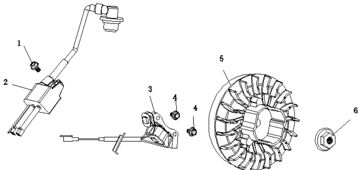
HPG1600i2 フライホイール/イグニッションコイル (FLYWHEEL/IGNITION COIL ASSY)
